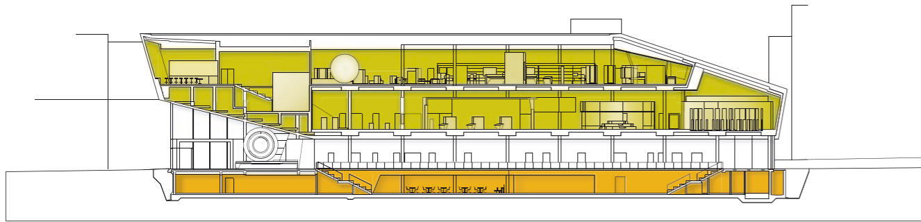
Längsschnitt, M 1:750
